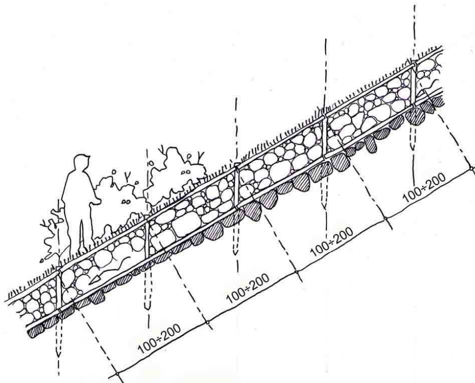
□ Profilo longitudinale
